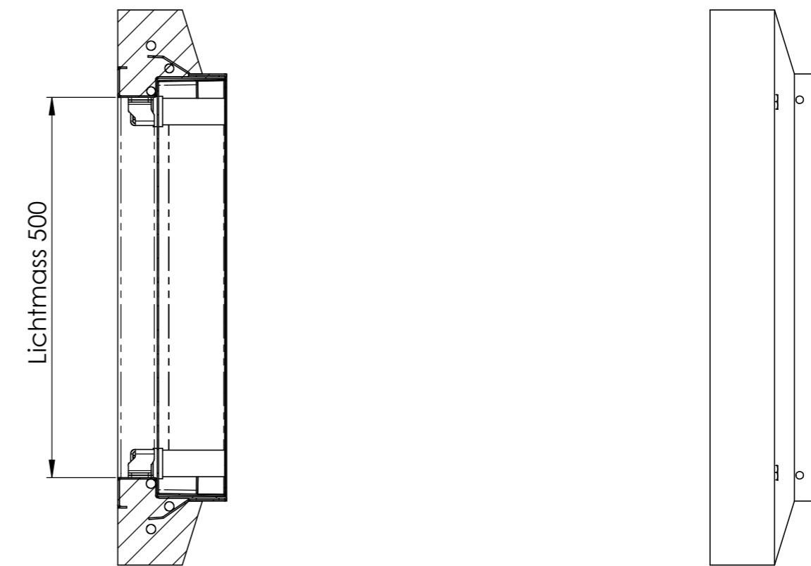
SCHNITT A-A MABSTAB 1 : 7
